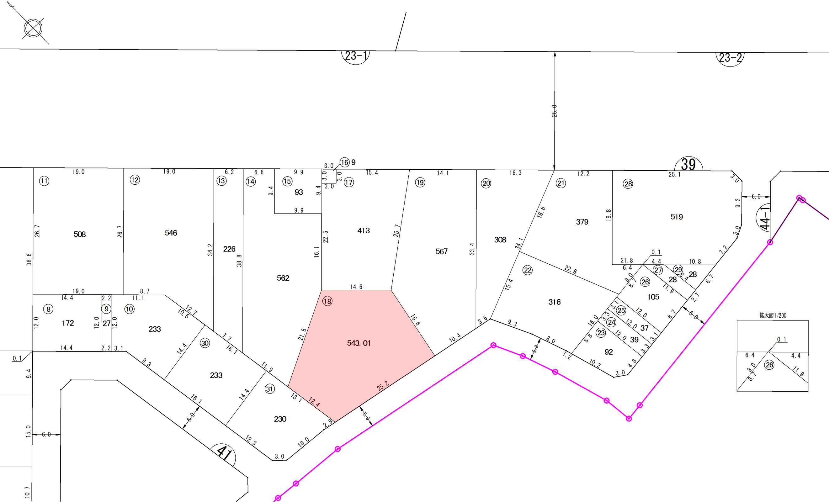
縮尺 1 : 500
