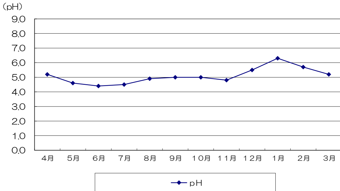
図 雨水のpHの経月推移
