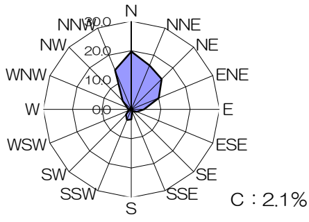
図 季節別風配図
