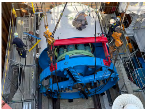
▲シールドマシンの組立
